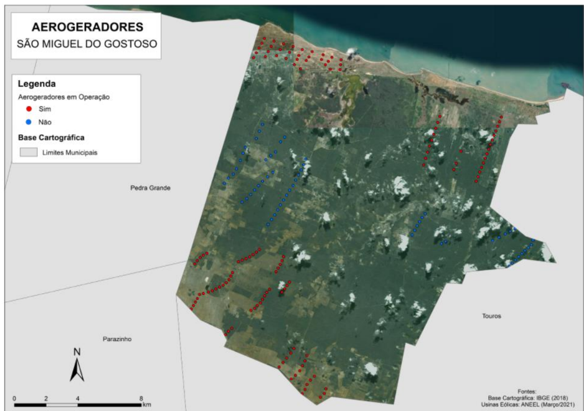
Figura 53: Uso do território de São Miguel do Gostoso pelo setor eólico, com a localização dos aerogeradores (em operação e ainda sem operar)
