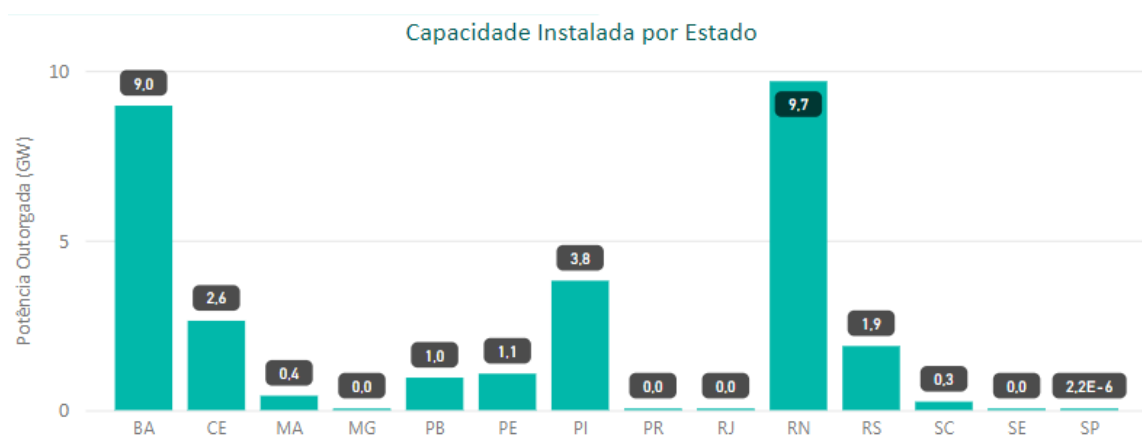
Figura 18: Capacidade instalada por estado
